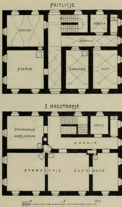
Župnišče. Tloris.
